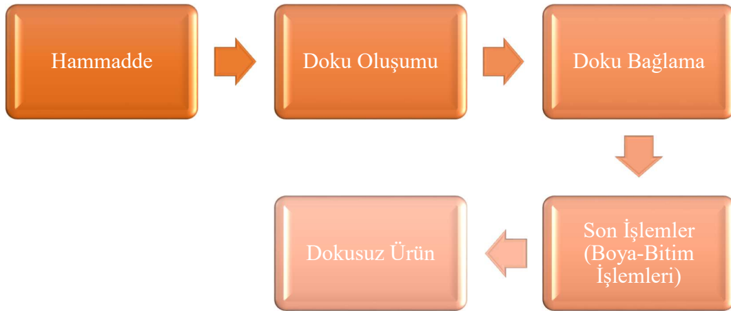
Şekil I.18. Dokusuz (Nonwoven) Ürün İmalatı İş Akış Şeması
