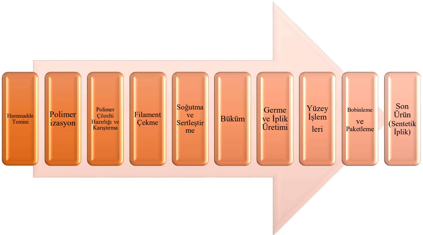
Şekil I.6. Sentetik İplik Üretimi İş Akış Şeması
